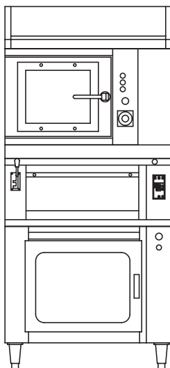
2 Topaze L04 + Rubis R4 + étuve + hotte + pieds + élévateur + enfourneur. 2 Topaze L04 + Rubis R4 + hood + proofer on feet + elevator + loader.
