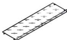
Полка стеклянная с ограничителем PA 100 PSFG 975x281x8
