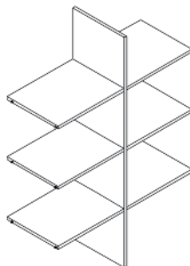
Накопитель на 8 ячеек PA 100150 N8 975x374x1455
