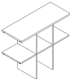
Накопитель на 6 ячеек PA 85100 N6 975x394x825
