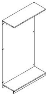
Стеллаж (корпус) PA 50120 C 1200x450x2200
